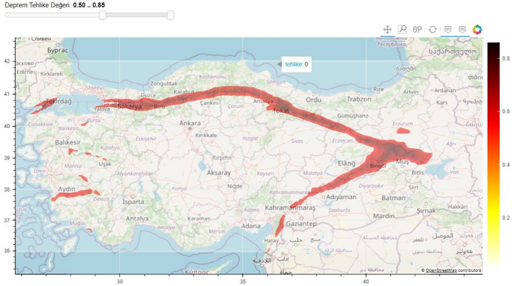
Şekil 1: Türkiye'nin 0.50-0.85 g ivme Değerli Arasındaki En Riskli Alanlarını Gösterir Harita
