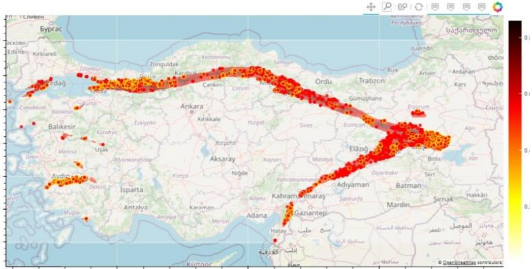
Şekil 2: Türkiye'nin 0.50-0.85g ivme Değerli Arasındaki En Riskli Alanları İçinde Kalan Okulların Lokasyonu Gösterir Harita
